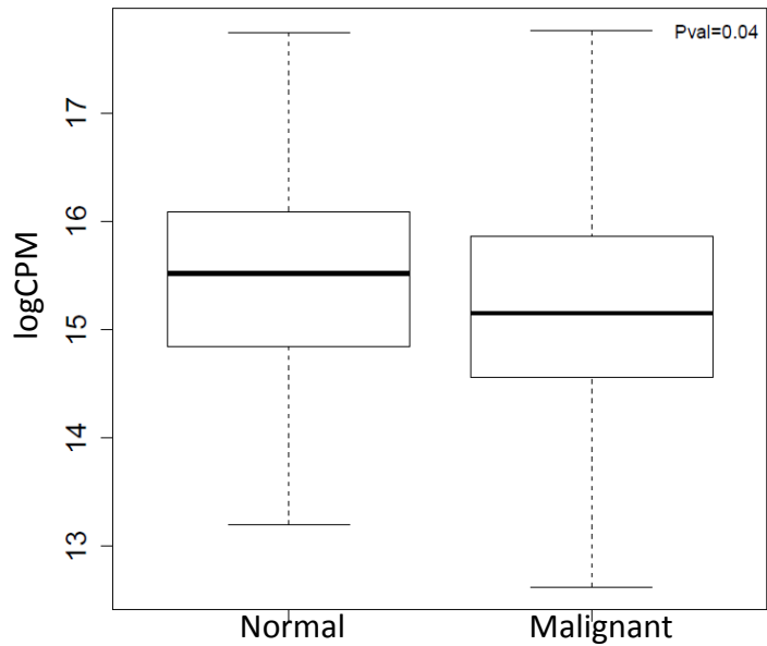
TCGA miRNA 148a-3p
