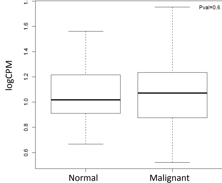
GSE51908 miRNA 374a-5p
