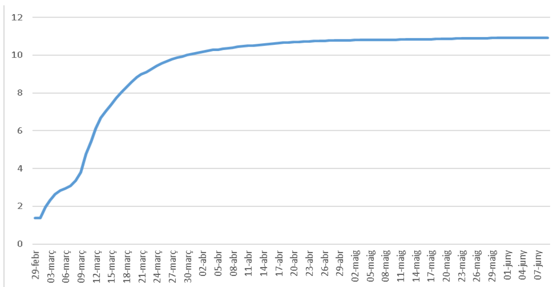
Figura 3. Curva temporal de casos confirmados acumulados de la COVID-19 en Cataluña. Escala logarítmica.
