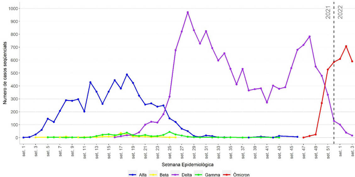
Figura 4. Nombre de casos de SARS-CoV-2 segons VOC i setmana. Catalunya, 4 de gener 2021 - 23 de gener de 2022
