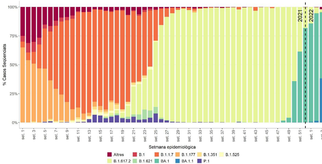
Figura 3. Percentatge dels casos dels 10 llinatges i variants del SARS-CoV-2 més freqüents per setmana. Catalunya, 4 de gener 2021 - 23 de gener de 2022
