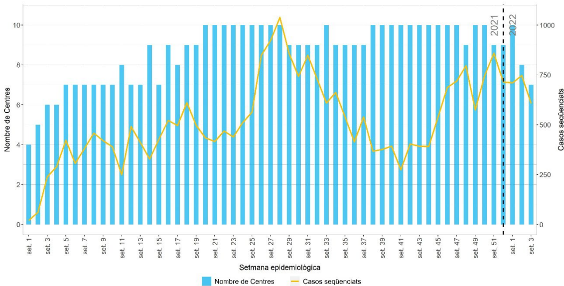
Figura 1. Nombre de casos de SARS-CoV-2 seqüenciats per nombre de centres declarants. Catalunya, 4 de gener 2021 - 23 de gener de 2022
